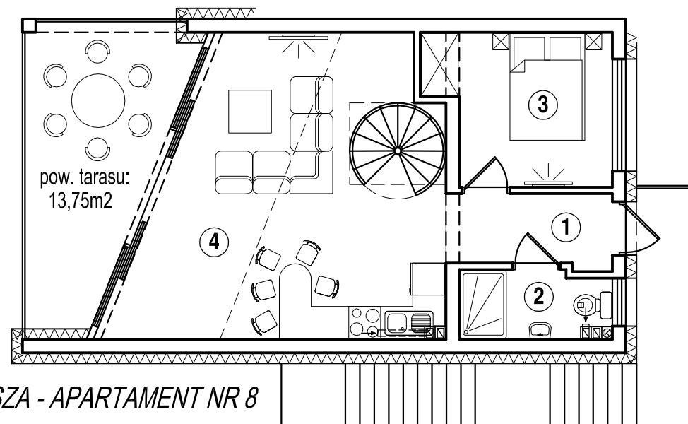
RZUT ANTRESOLI - APARTAMENT NR 8
