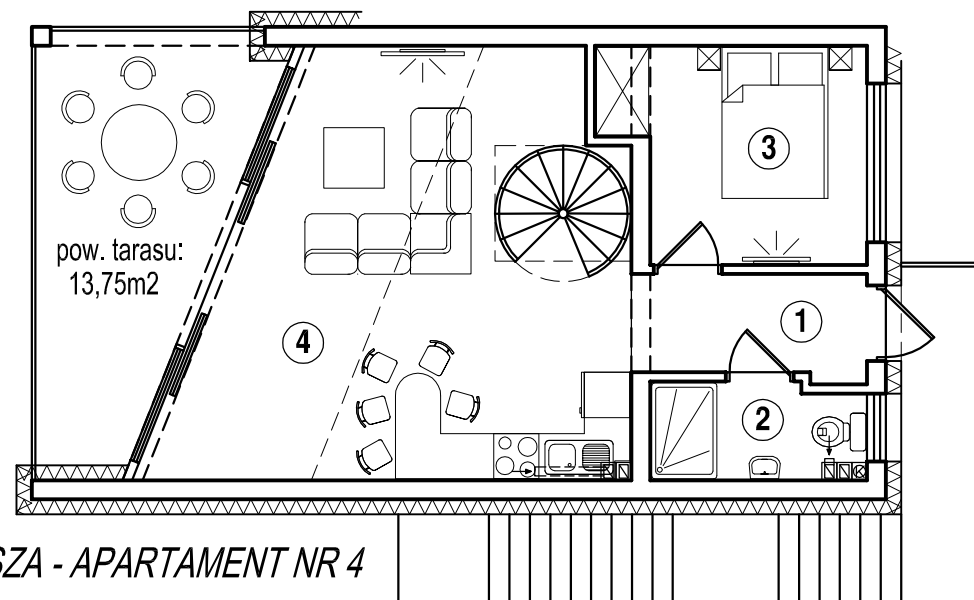
RZUT ANTRESOLI - APARTAMENT NR 4
